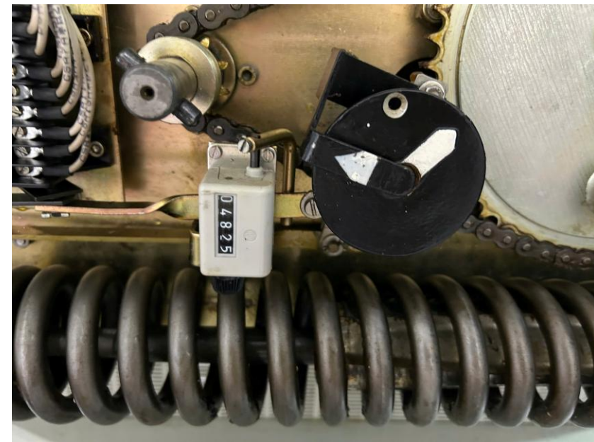
VI.6.d - Số lần đóng/cắt máy cắt 943
