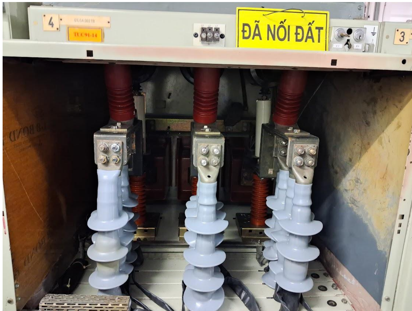
VI.8.b - Bên trong tủ DNE TUC91-14
