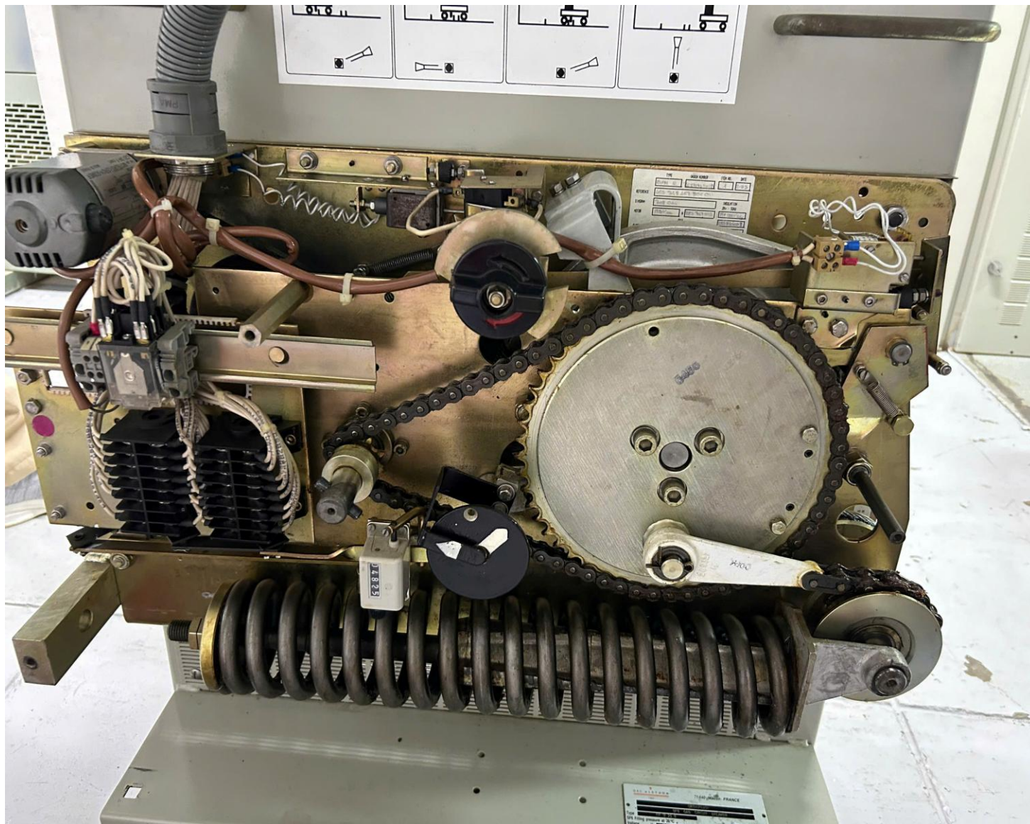
VI.6.c - Chi tiết máy cắt 943
