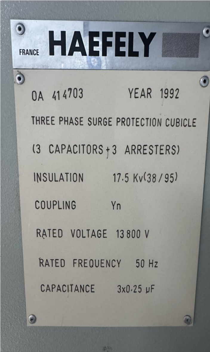
VI.9.c - Thông số tủ chống sét
