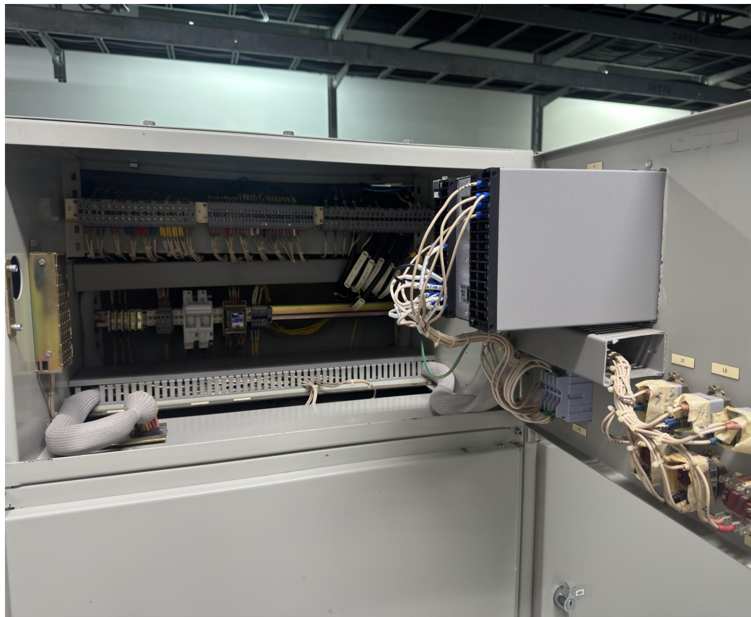
VI.5.b Bên trong tủ điều khiển máy cắt 943
